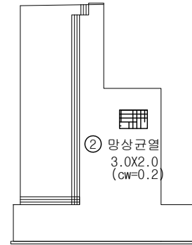
날개벽(우측)
